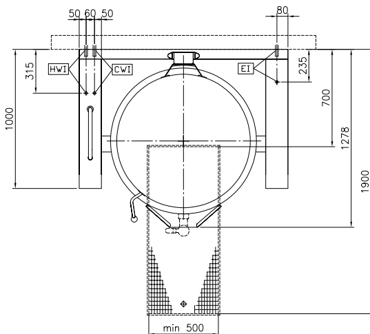
Boven aanzicht
